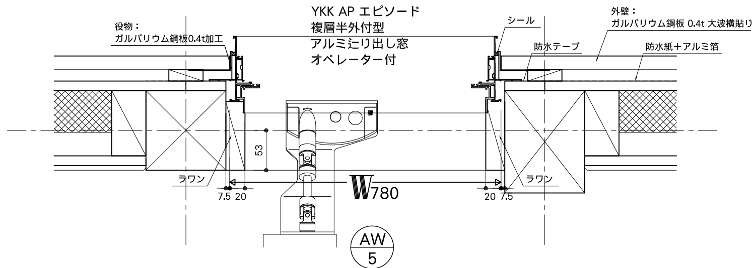
YKK AP エピソード 複層半外付型 アルミ引き出し窓 オペレーター付
