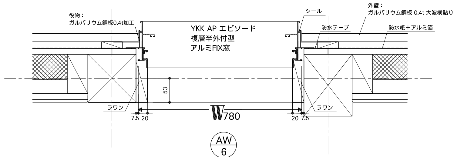
YKK AP エピソード 複層半外付型 アルミFIX窓
