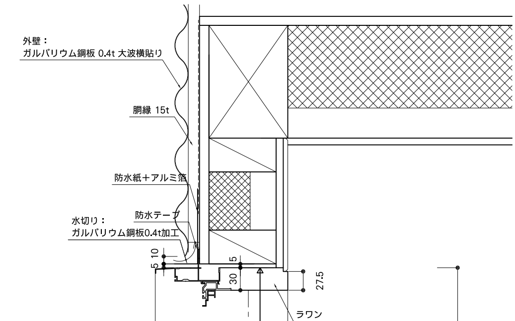
YKK AP エピソード 複層半外付型 アルミ引き出し窓 オペレーター付
