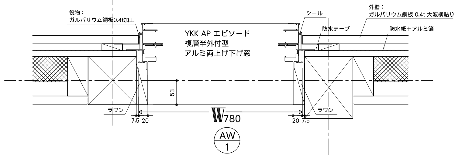
YKK AP エピソード 複層半外付型 アルミ両上げ下げ窓
