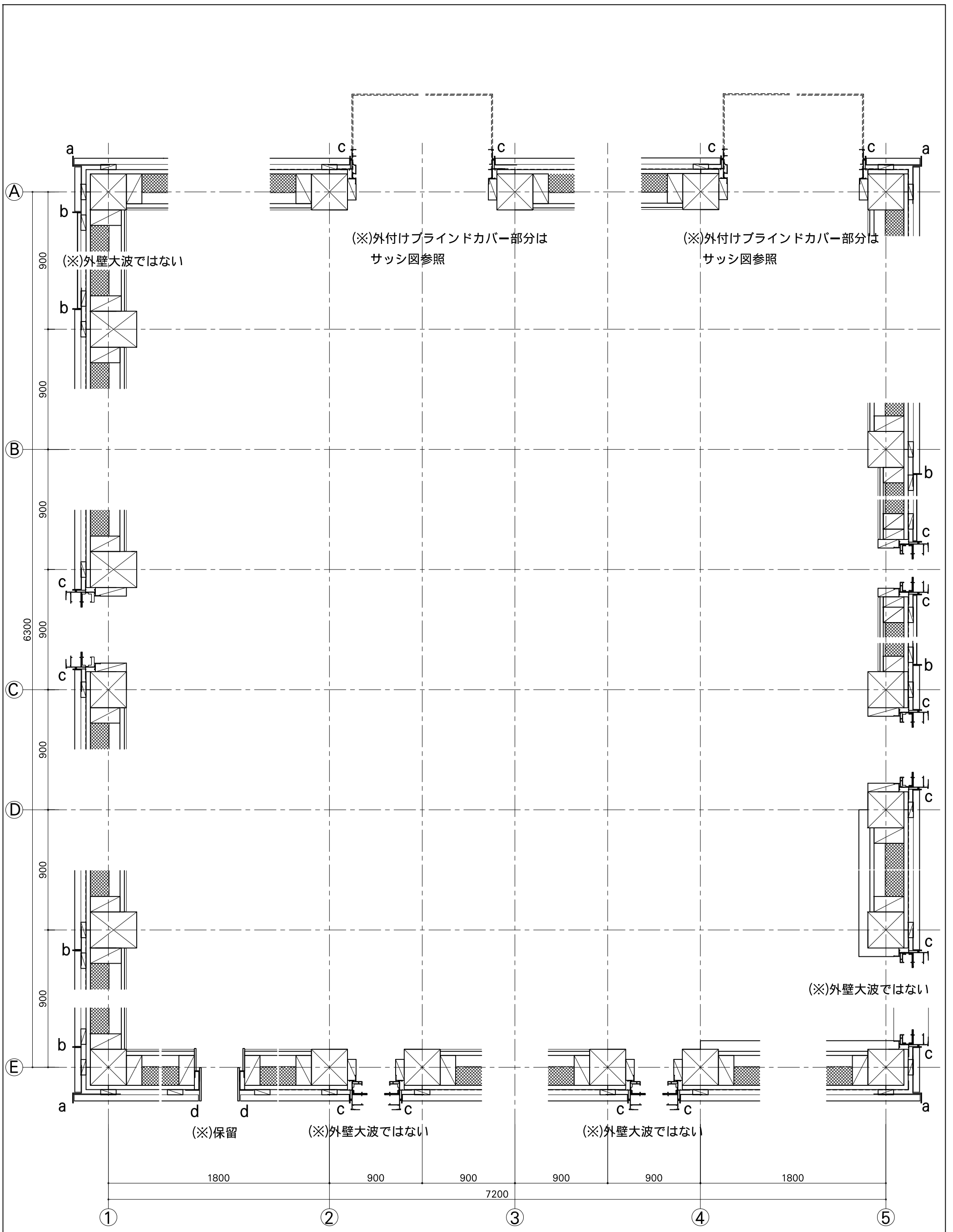
平面図A
