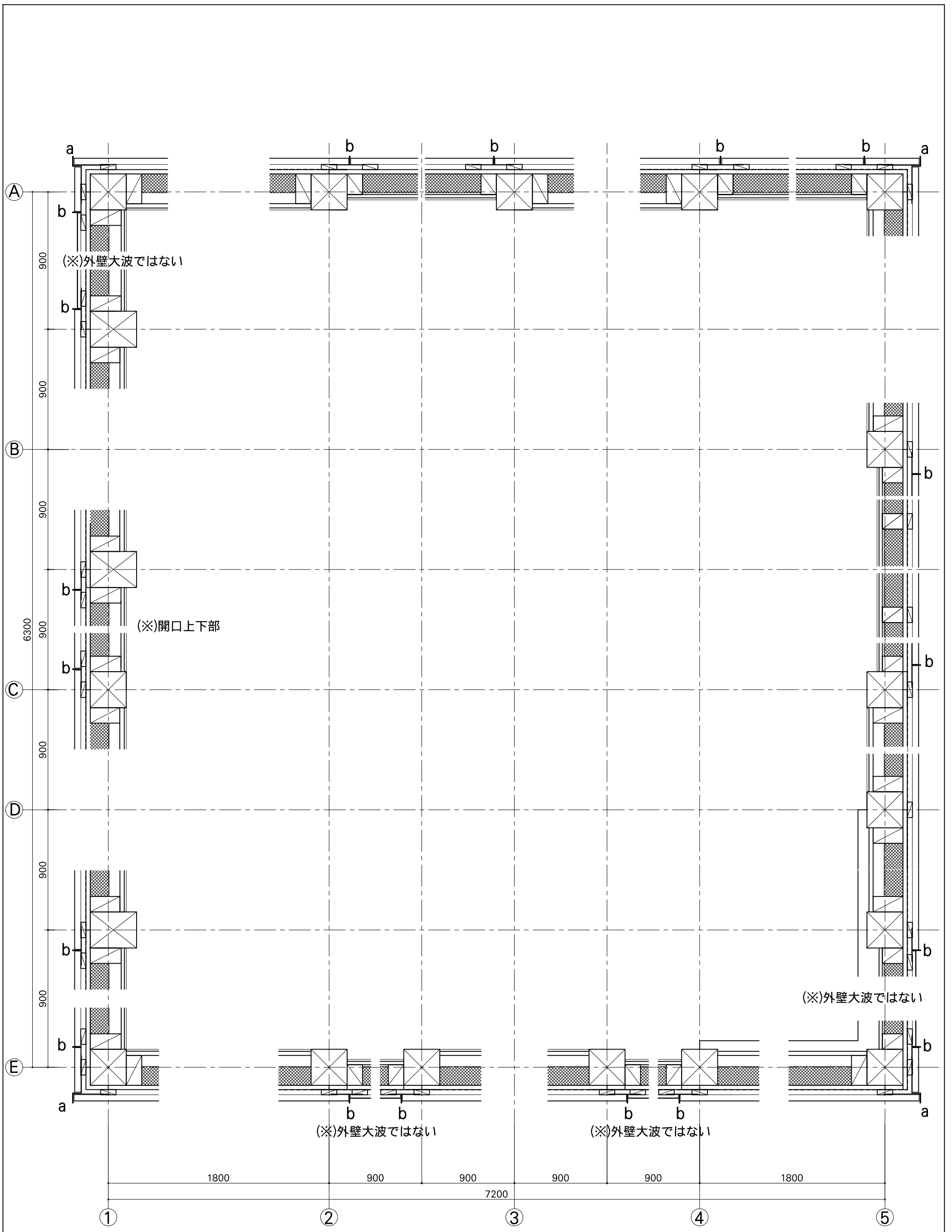
平面図B
