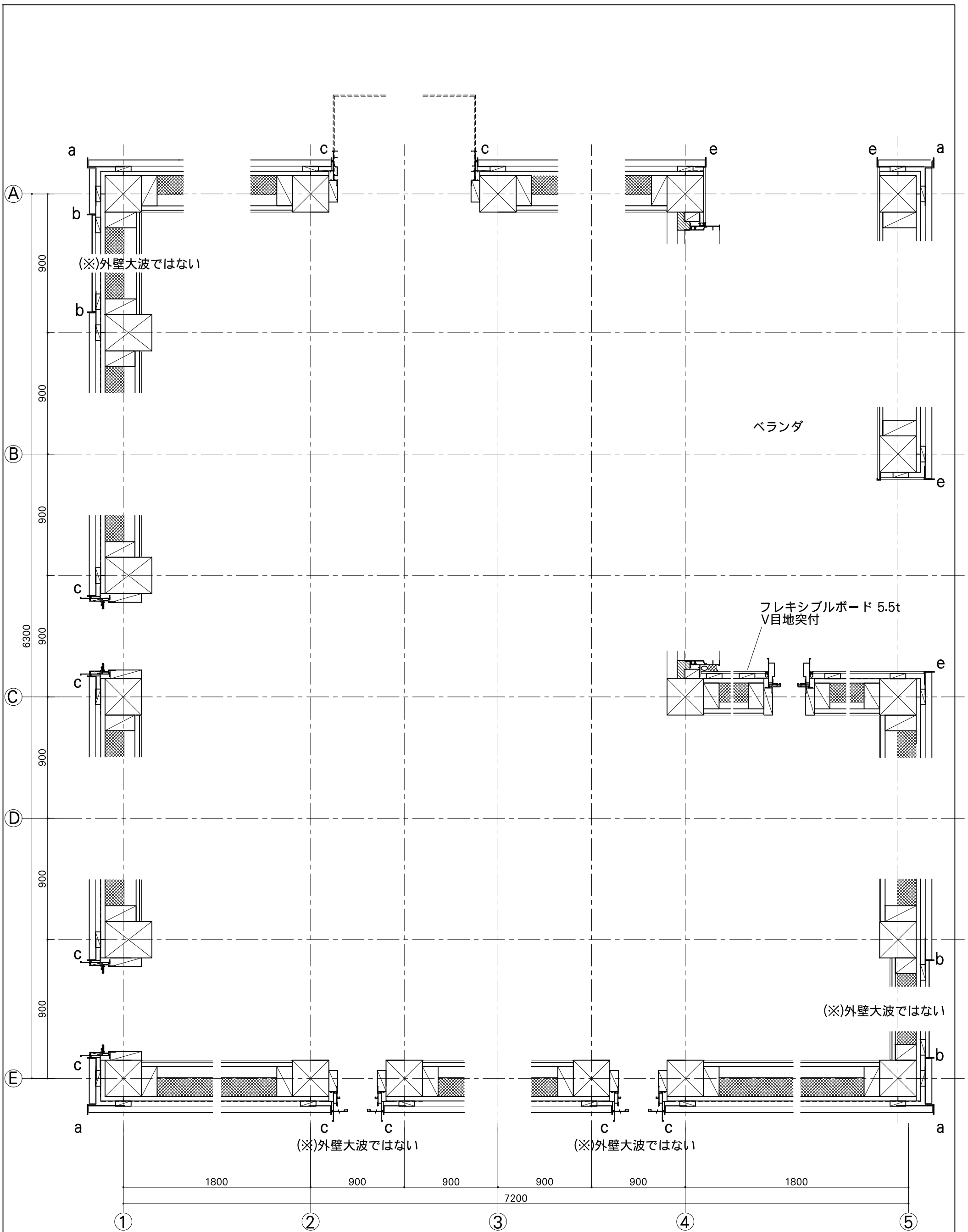
平面図C
