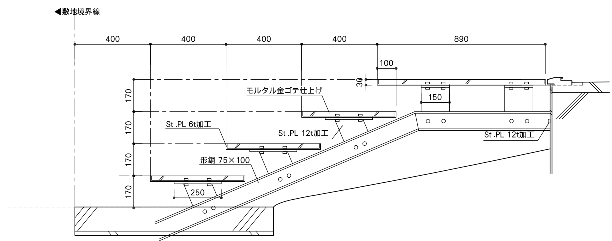
断面図
