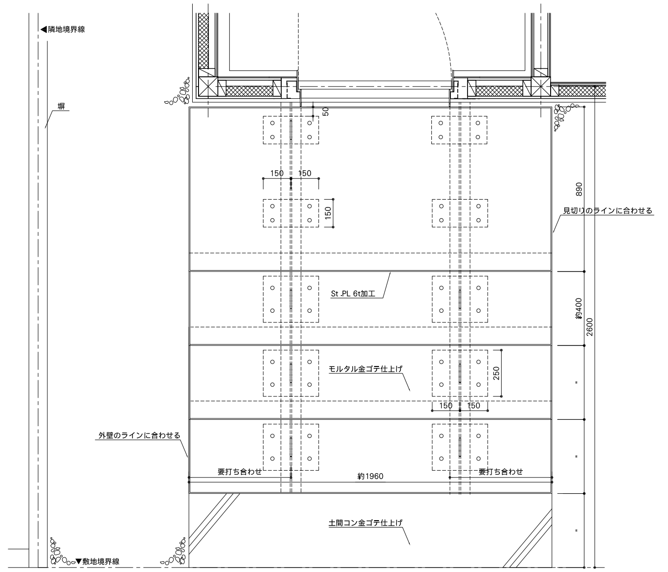
平面図
