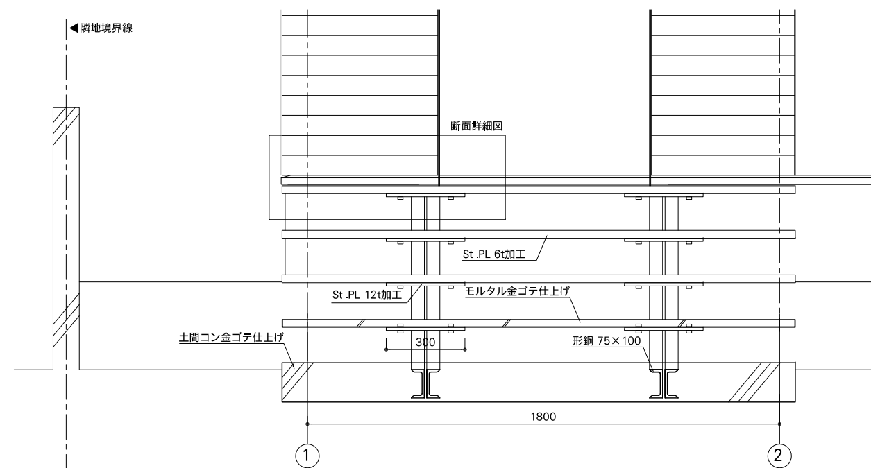
立面図
