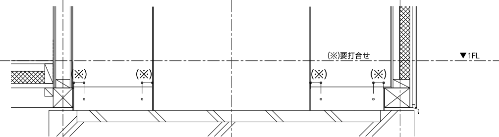
断面図 C
