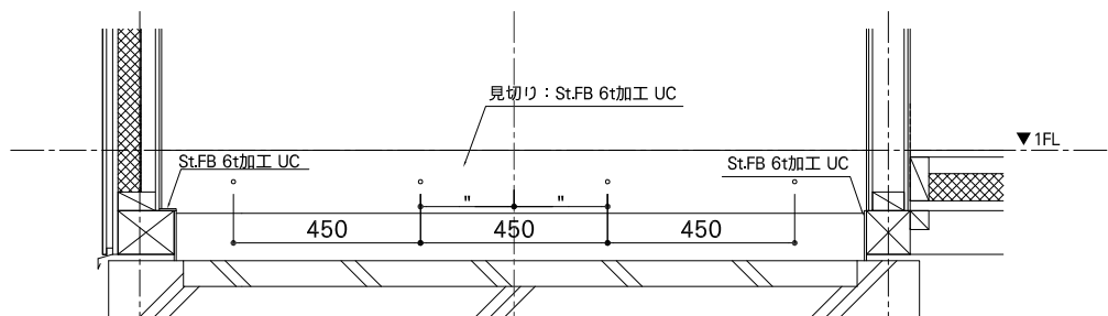
断面図 A
