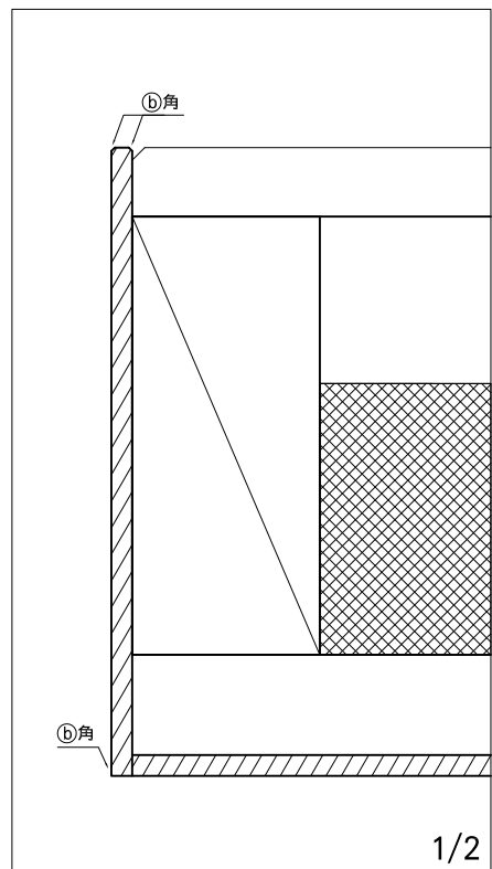
詳細断面図 c 1/5
