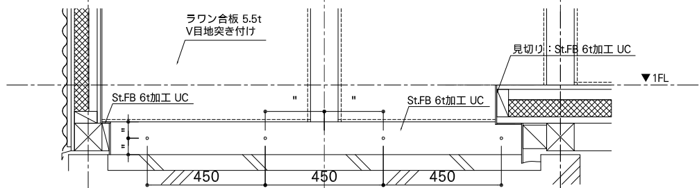
断面図 B
