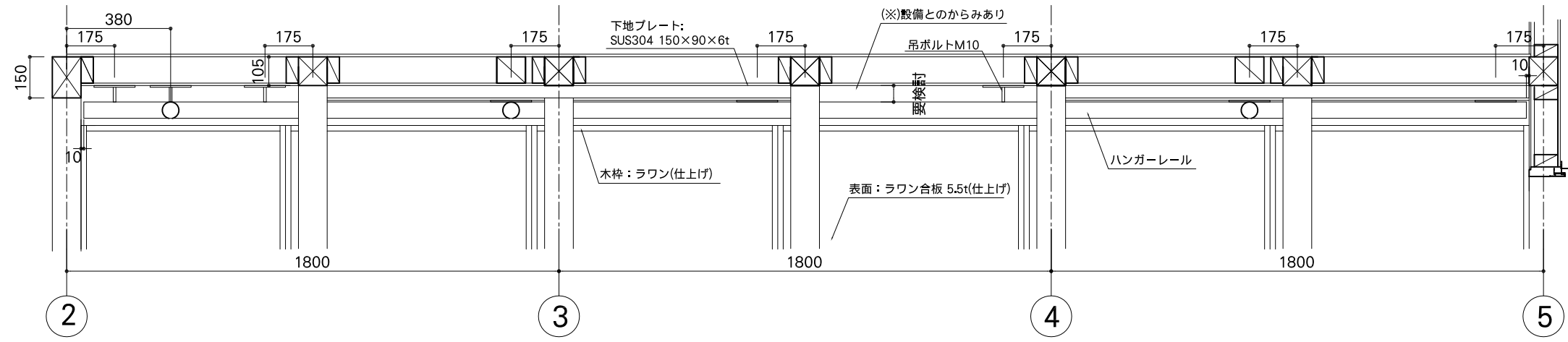
P断面図
