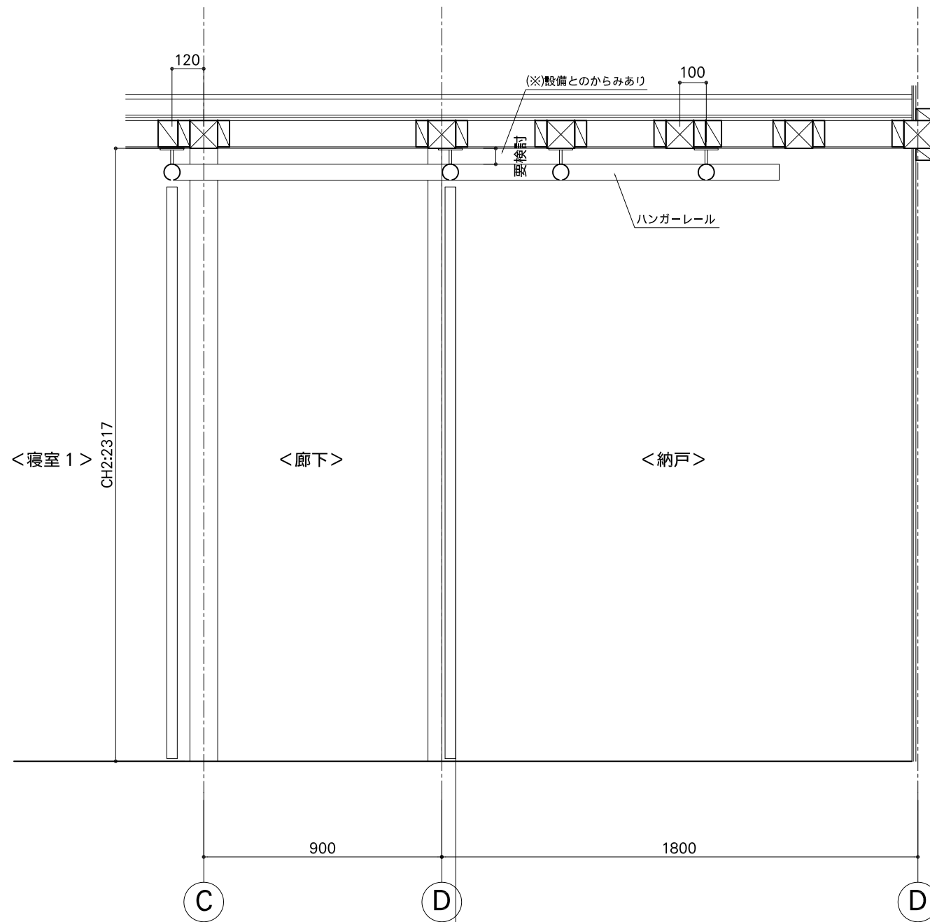
S1断面図
