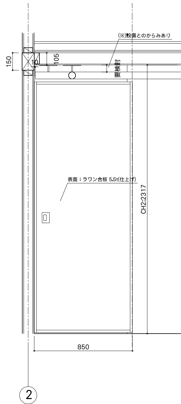
R断面図
