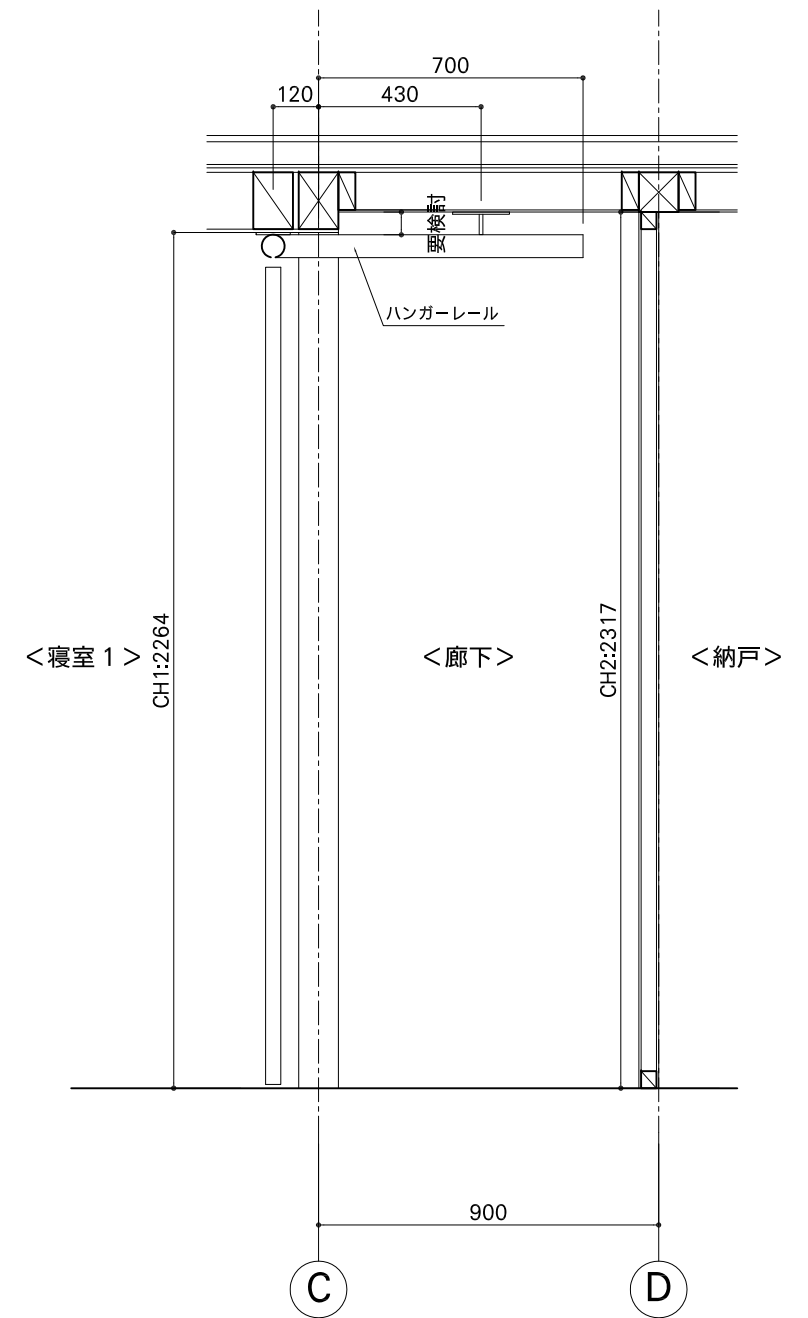
S2断面図
