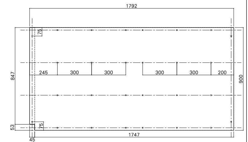
合板詳細図
