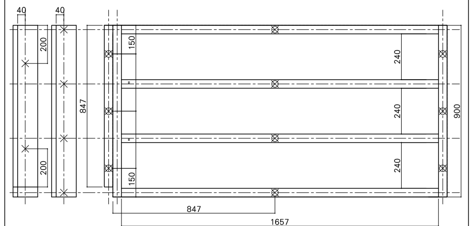
根太詳細図
