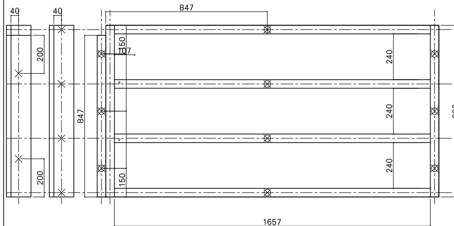
根太詳細図
