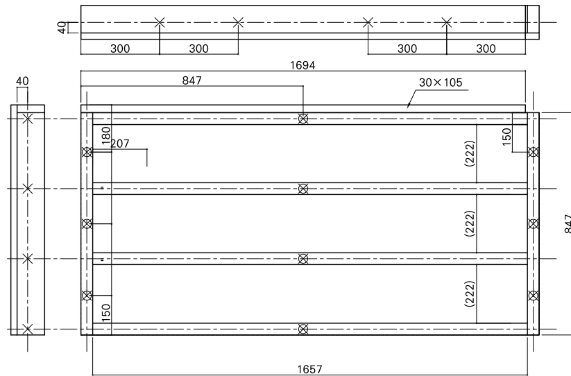
根太詳細図
