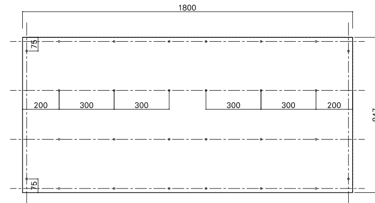
合板詳細図
