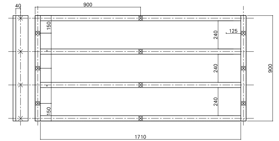
根太詳細図
