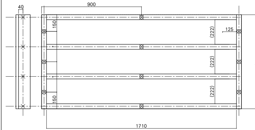
根太詳細図
