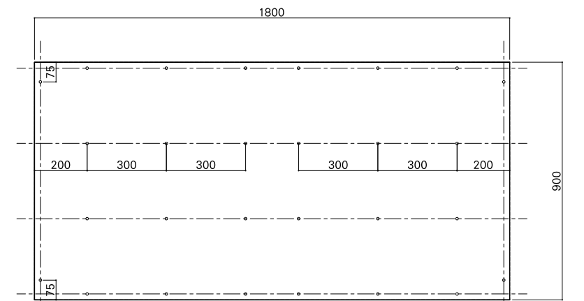
合板詳細図
