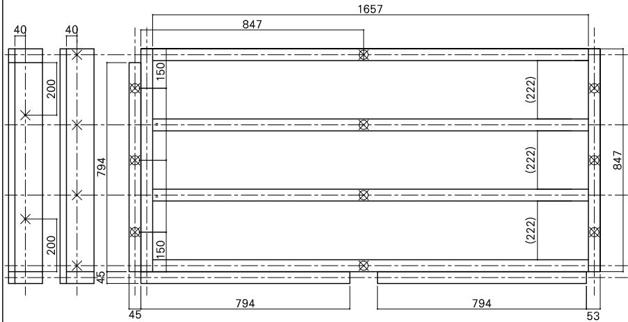
根太詳細図
