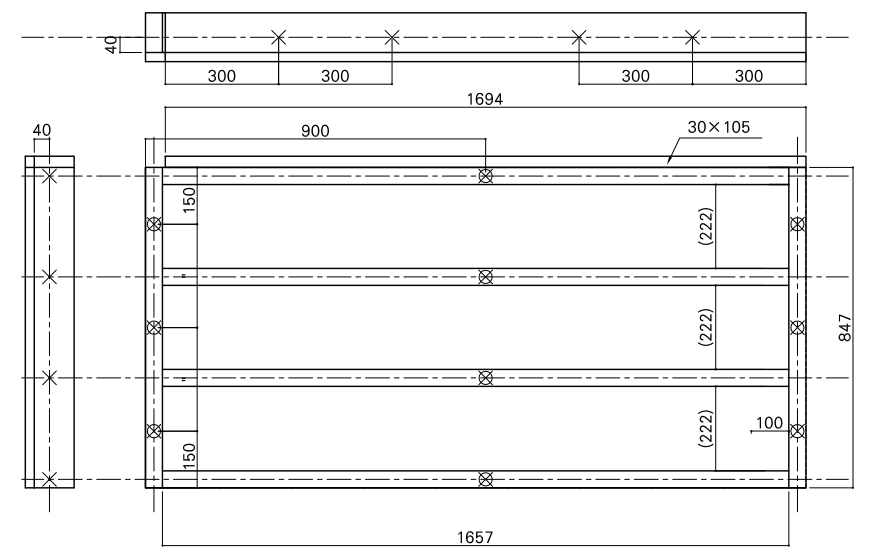
根太詳細図
