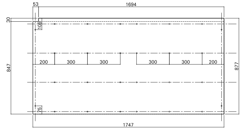
合板詳細図
