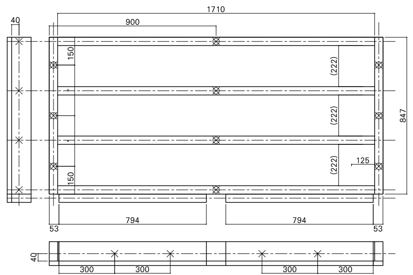
根太詳細図
