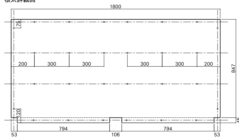
合板詳細図
