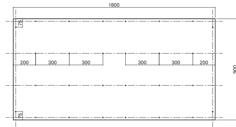
合板詳細図
