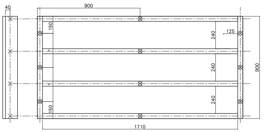
根太詳細図
