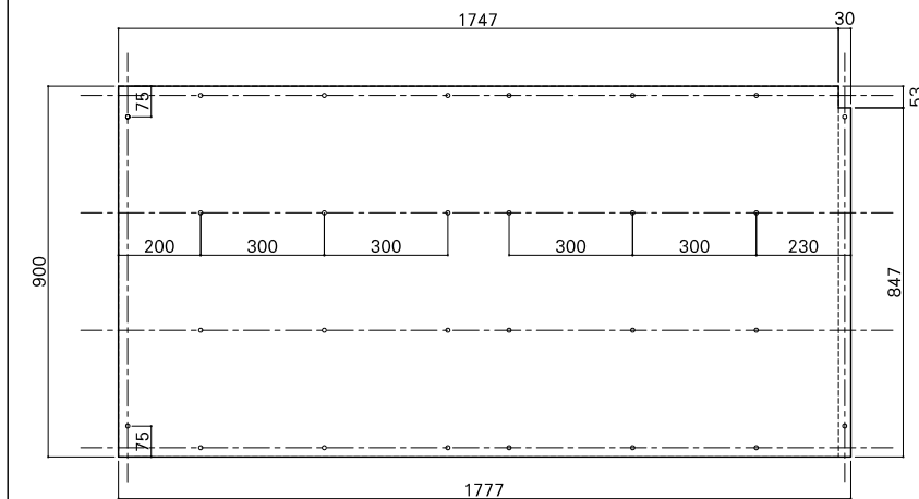
合板詳細図
