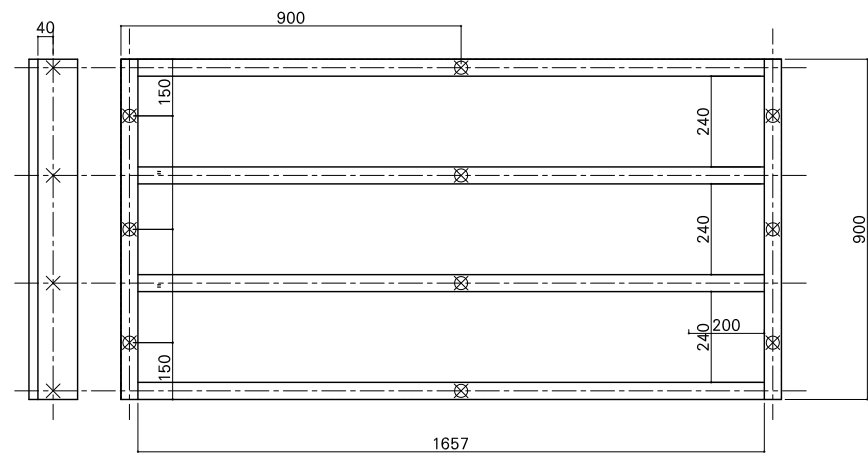
根太詳細図
