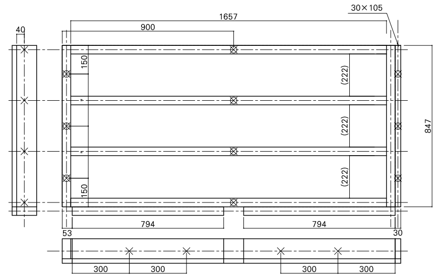
根太詳細図
