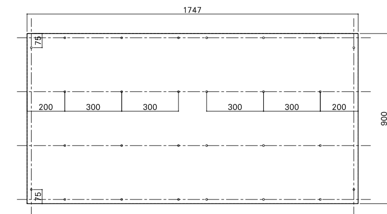
合板詳細図
