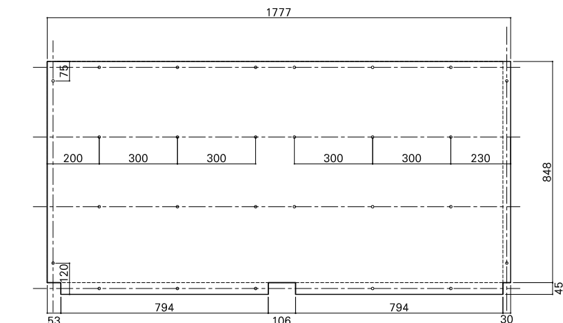
合板詳細図
