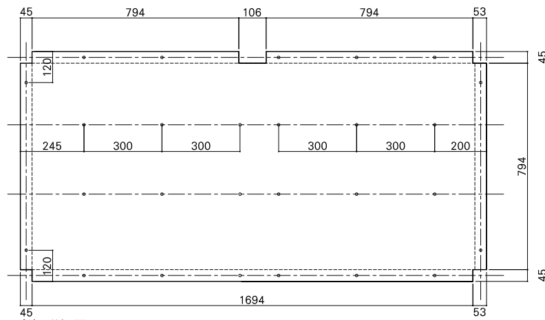
合板詳細図
