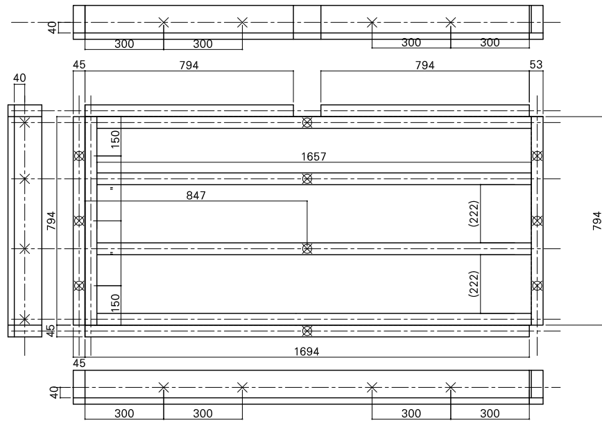
根太詳細図
