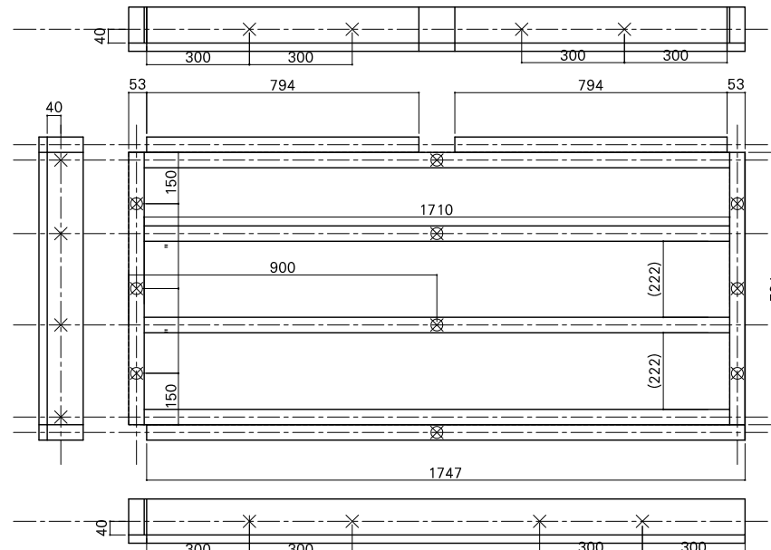
根太詳細図
