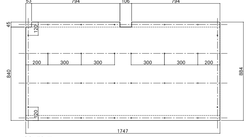
合板詳細図
