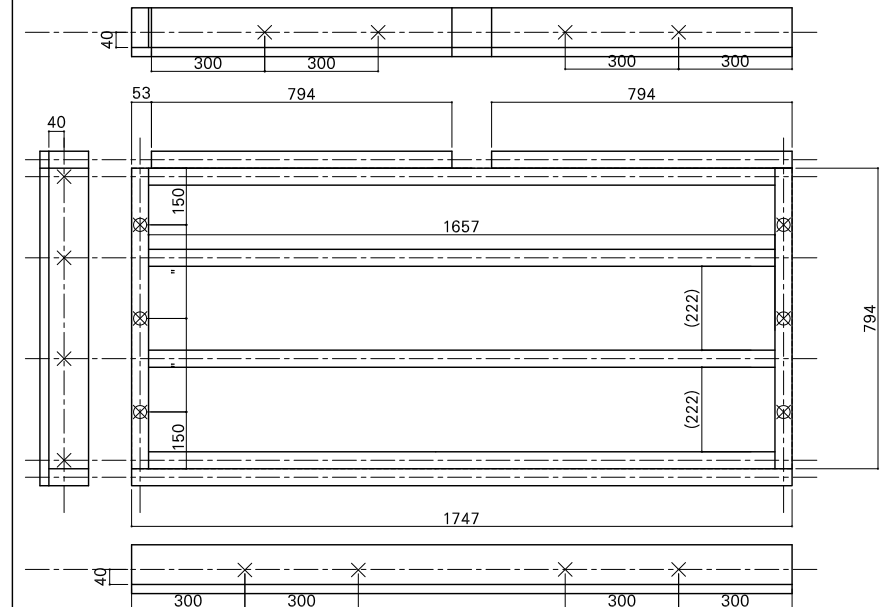
根太詳細図
