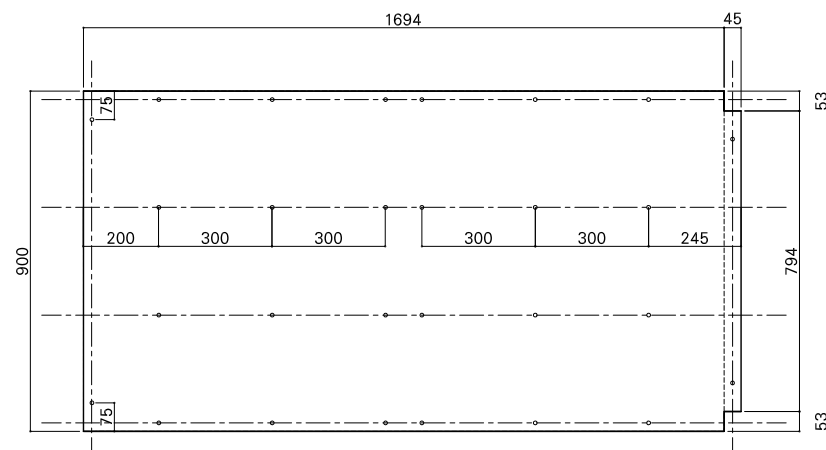
合板詳細図
