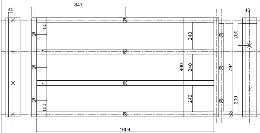
根太詳細図
