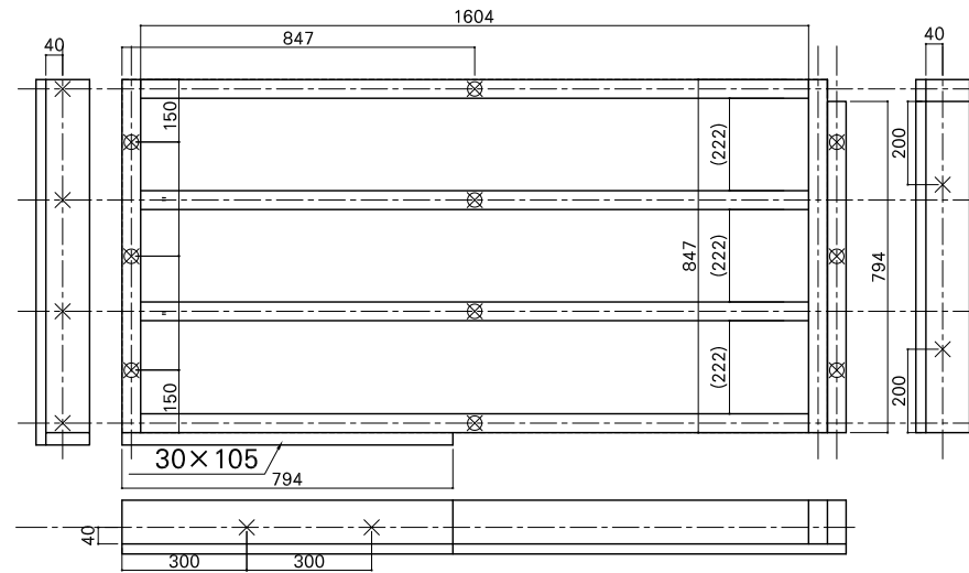
根太詳細図
