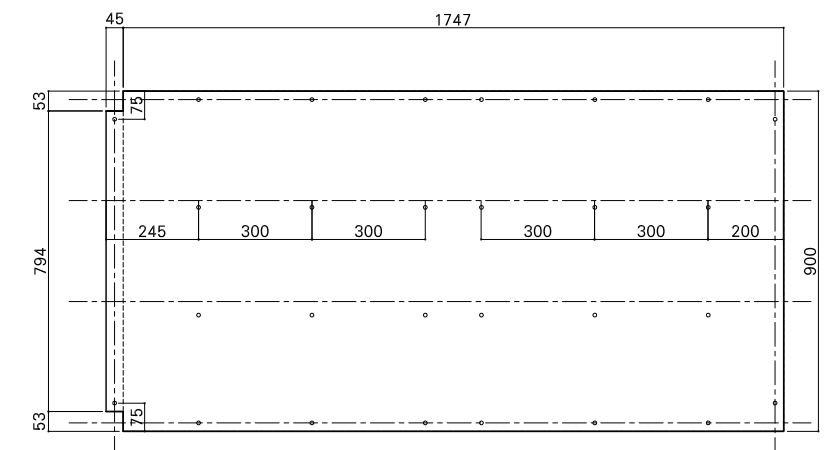
合板詳細図
