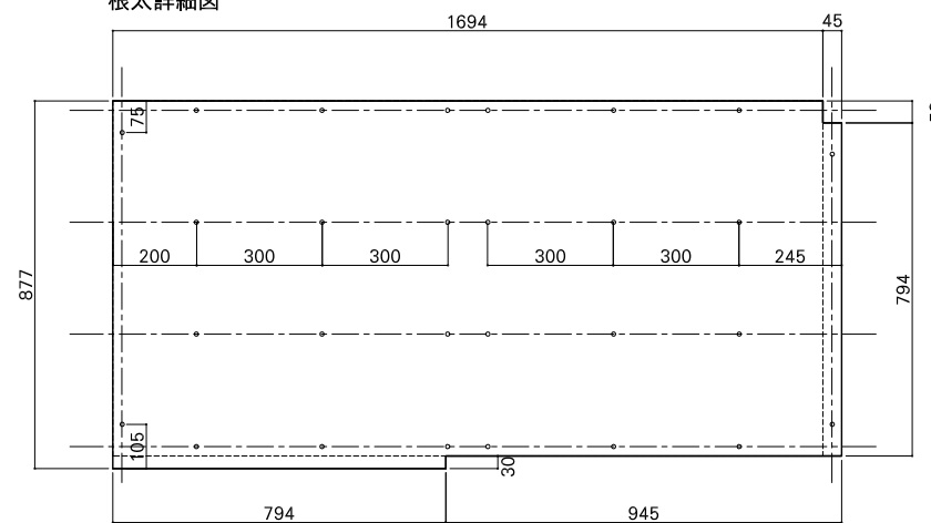
合板詳細図
