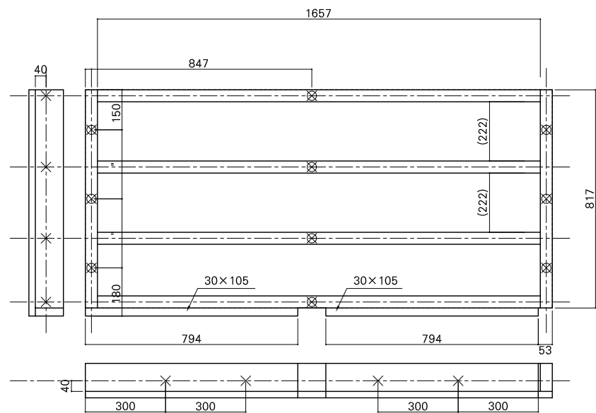
根太詳細図
