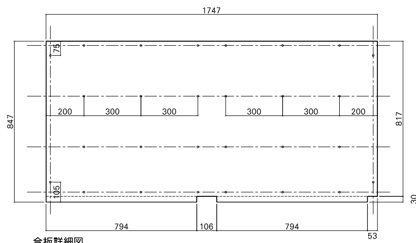
合板詳細図
