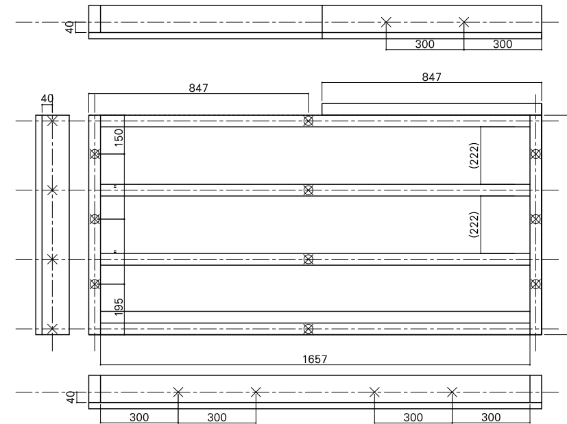
根太詳細図
