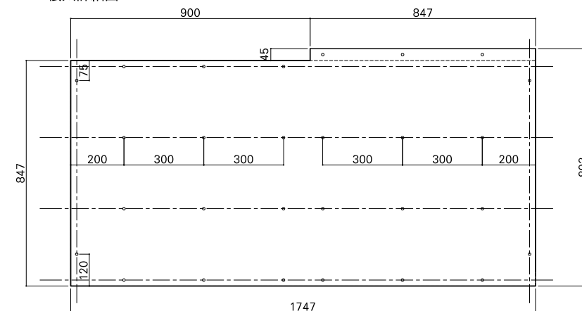
合板詳細図
