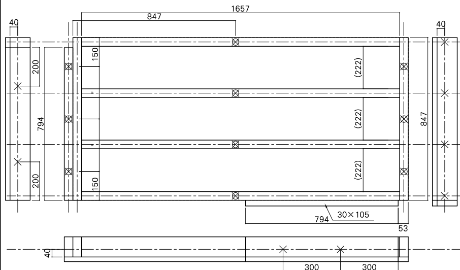
根太詳細図
