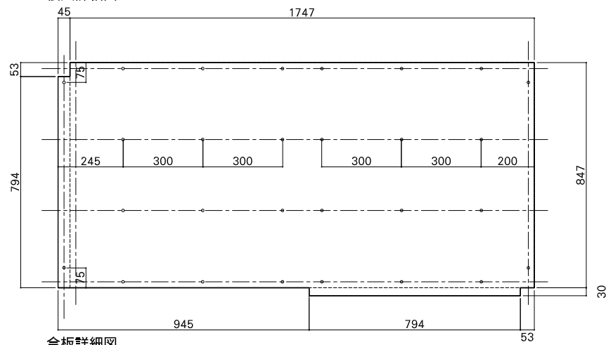
合板詳細図
