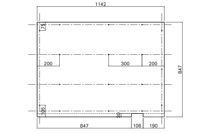
合板詳細図
