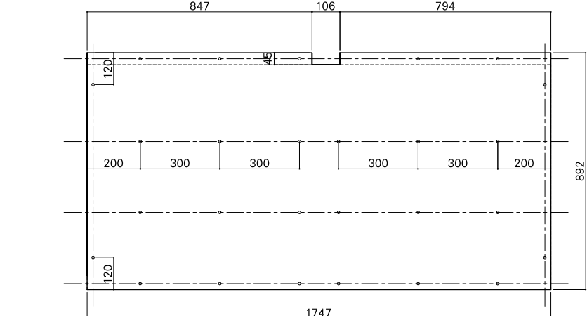
合板詳細図
