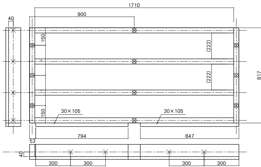
根太詳細図
