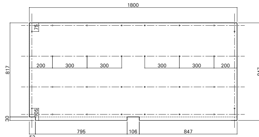
合板詳細図
