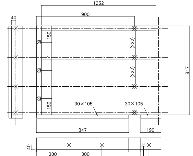
根太詳細図
