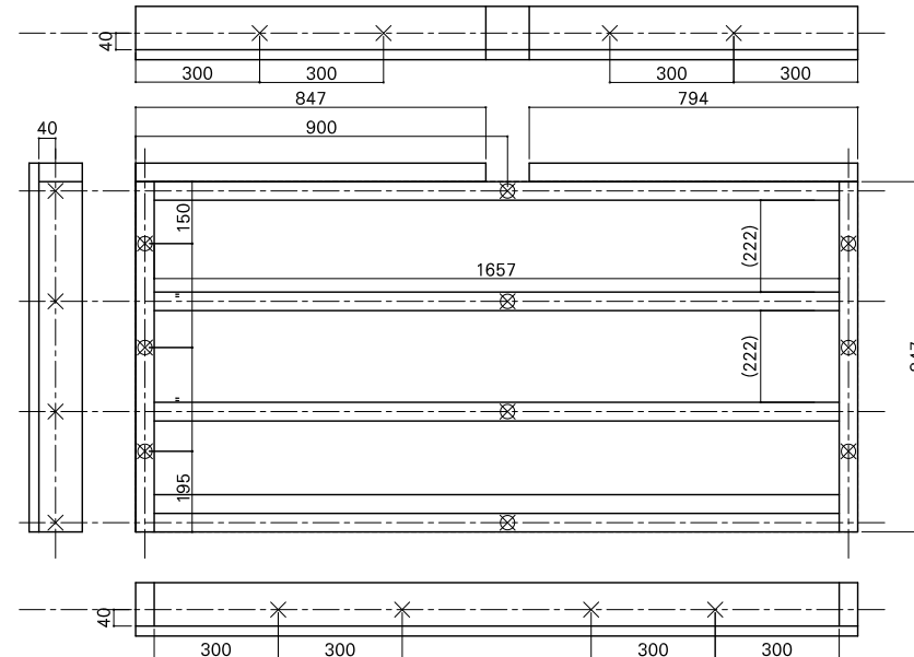
根太詳細図
