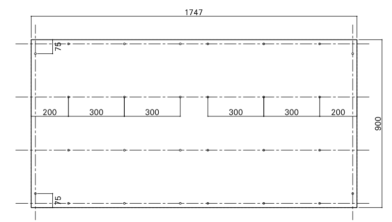
合板詳細図
