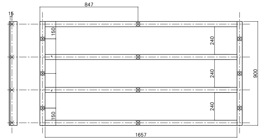
根太詳細図
