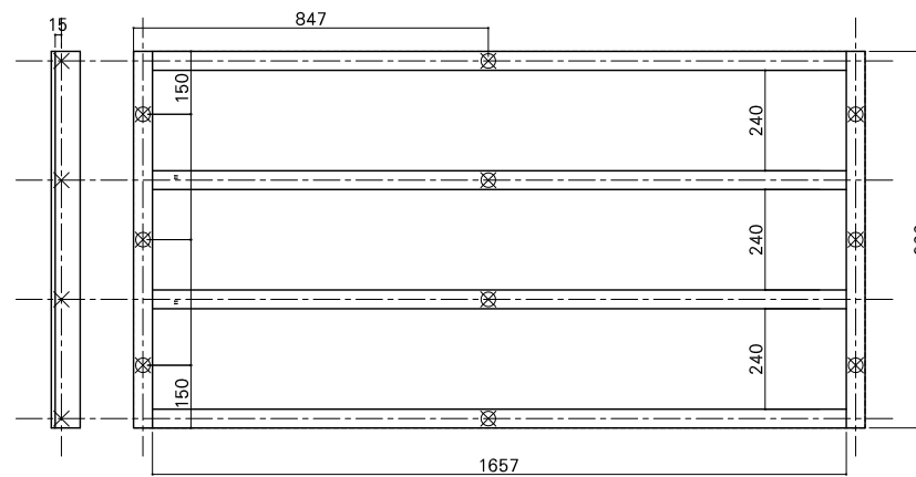
根太詳細図
