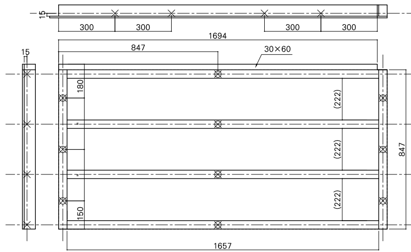
根太詳細図
