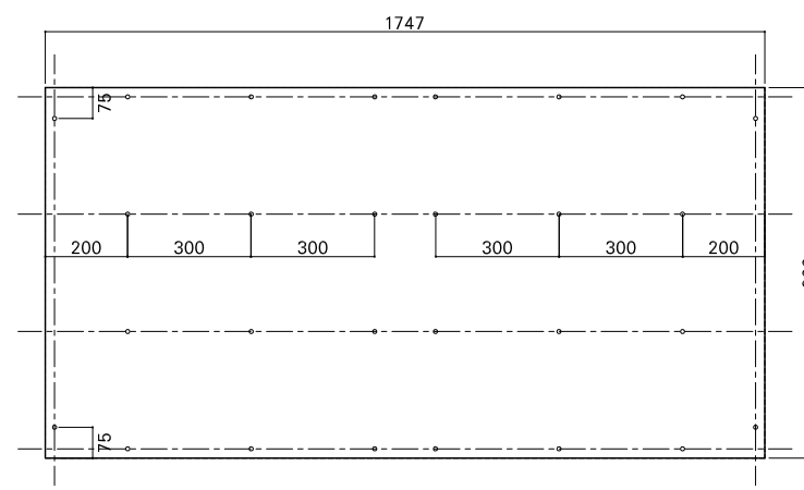
合板詳細図
