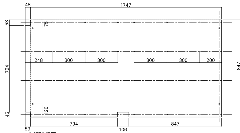
合板詳細図
