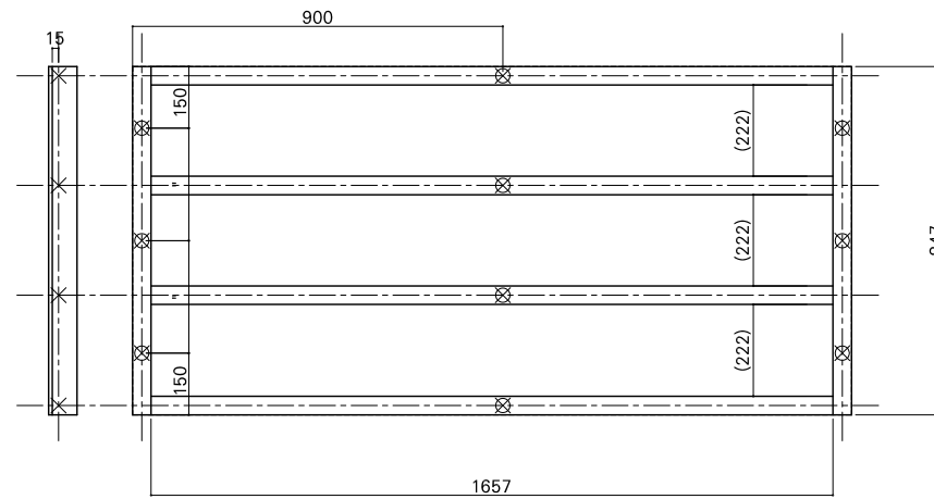
根太詳細図
