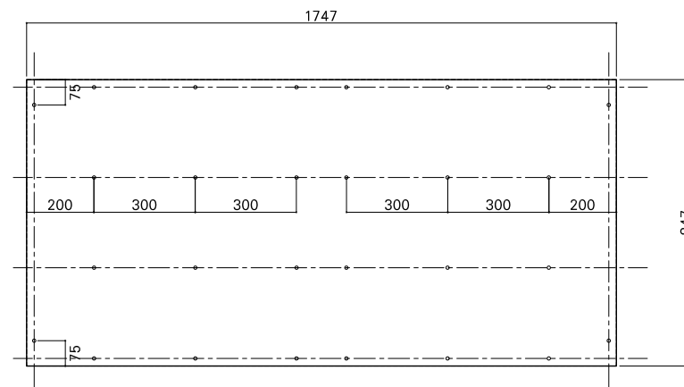
合板詳細図
