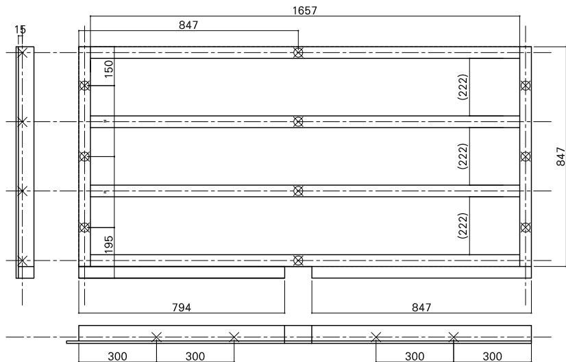
根太詳細図
