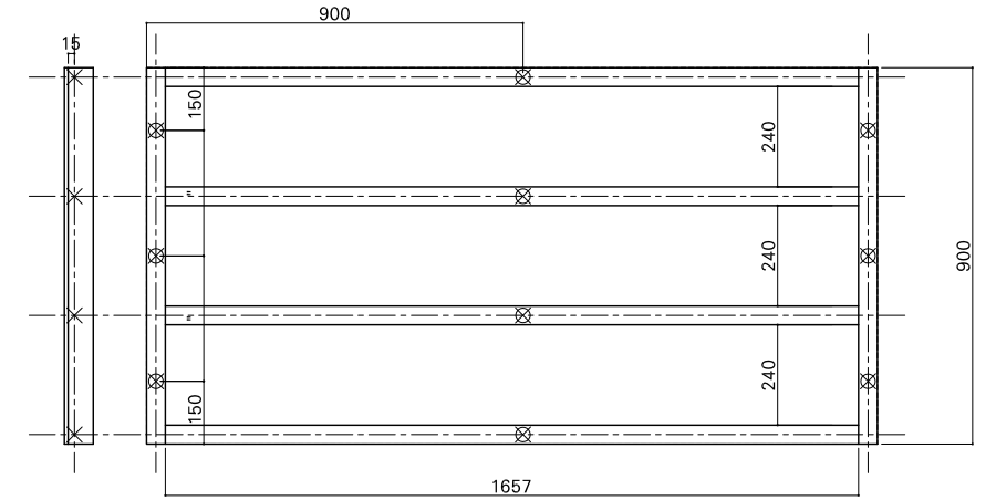
根太詳細図
