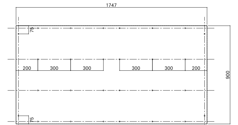
合板詳細図
