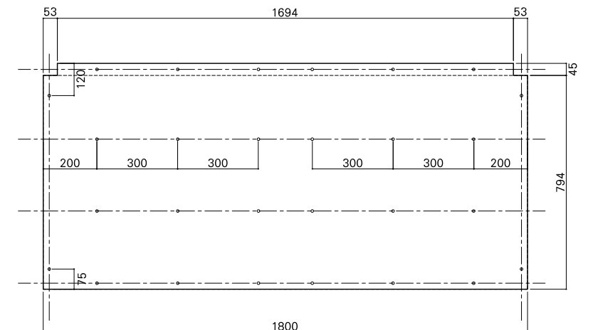
合板詳細図
