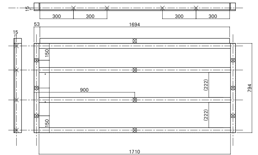
根太詳細図
