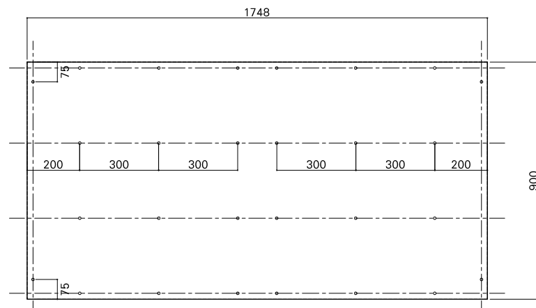
合板詳細図
