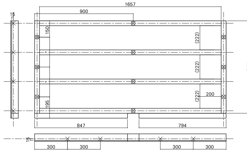
根太詳細図
