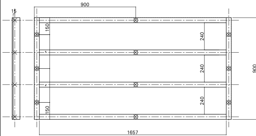
根太詳細図
