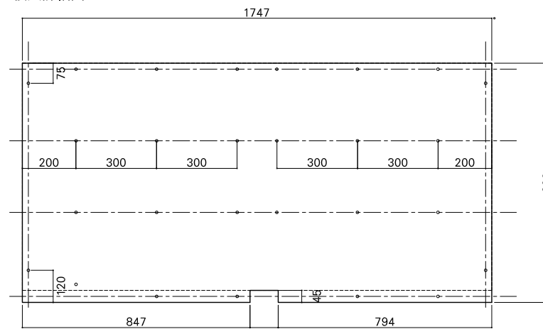
合板詳細図
