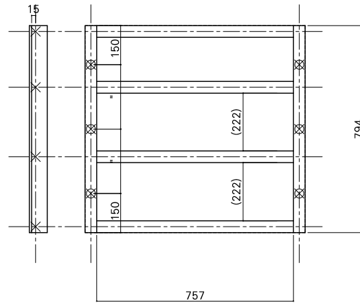
根太詳細図
