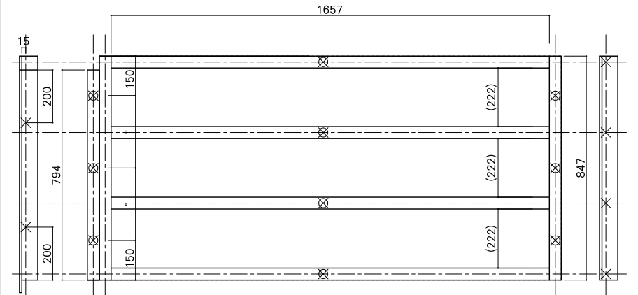
根太詳細図
