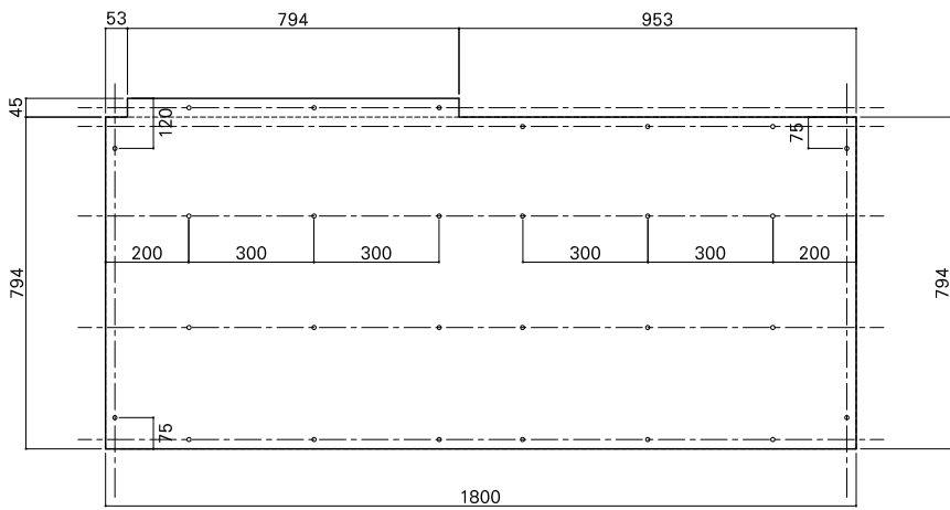
合板詳細図
