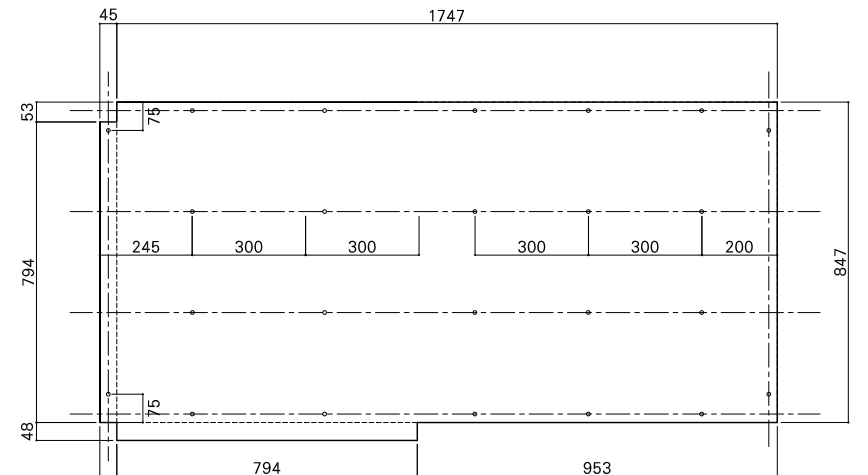
合板詳細図
