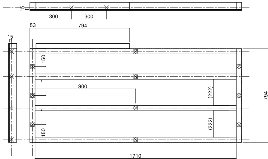
根太詳細図
