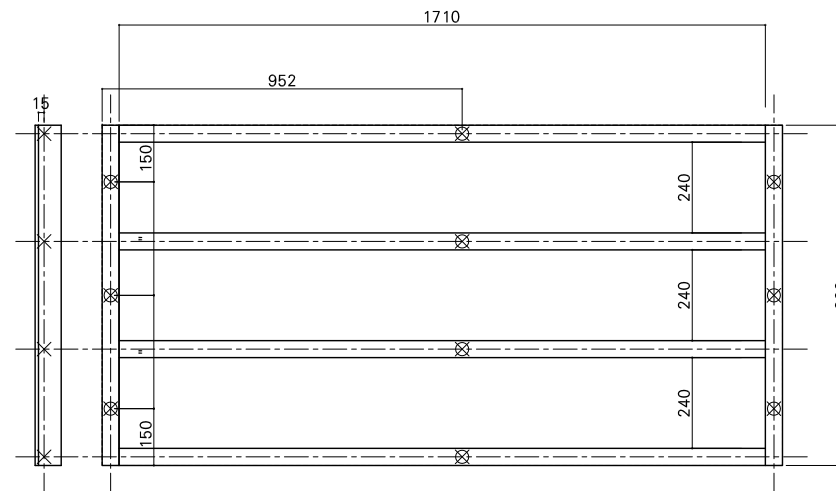
根太詳細図
