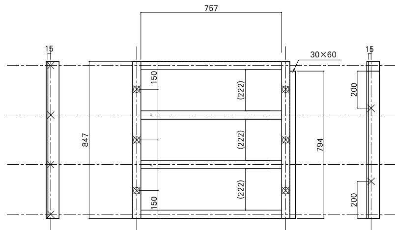
根太詳細図
