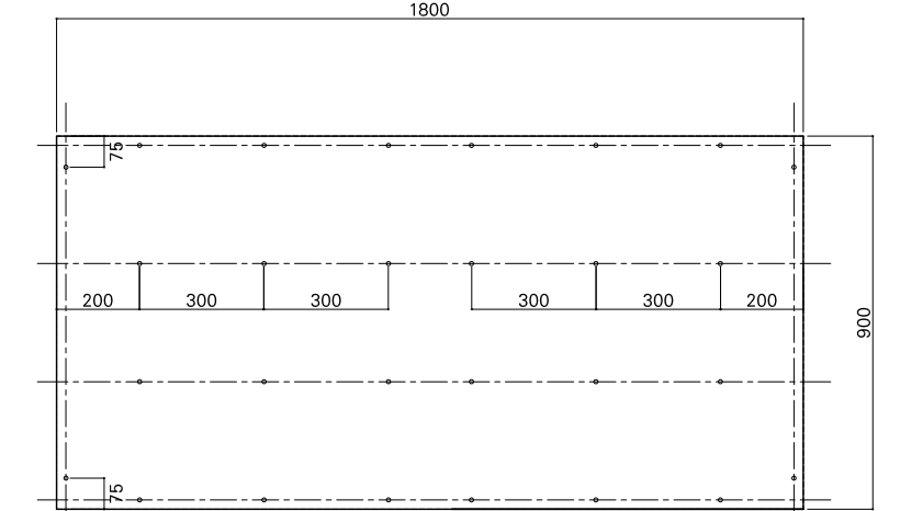
合板詳細図
