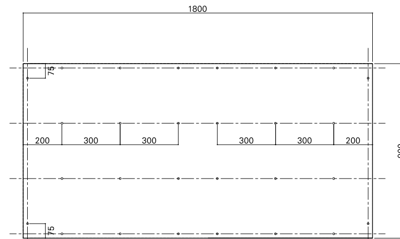
合板詳細図
