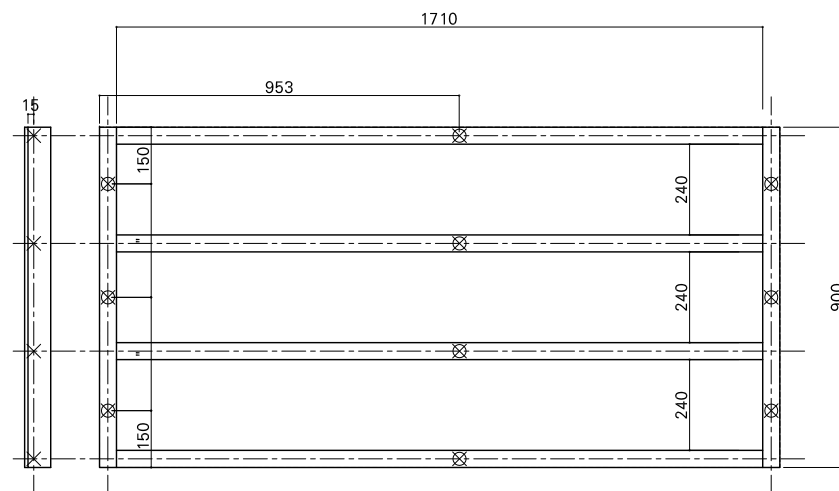
根太詳細図
