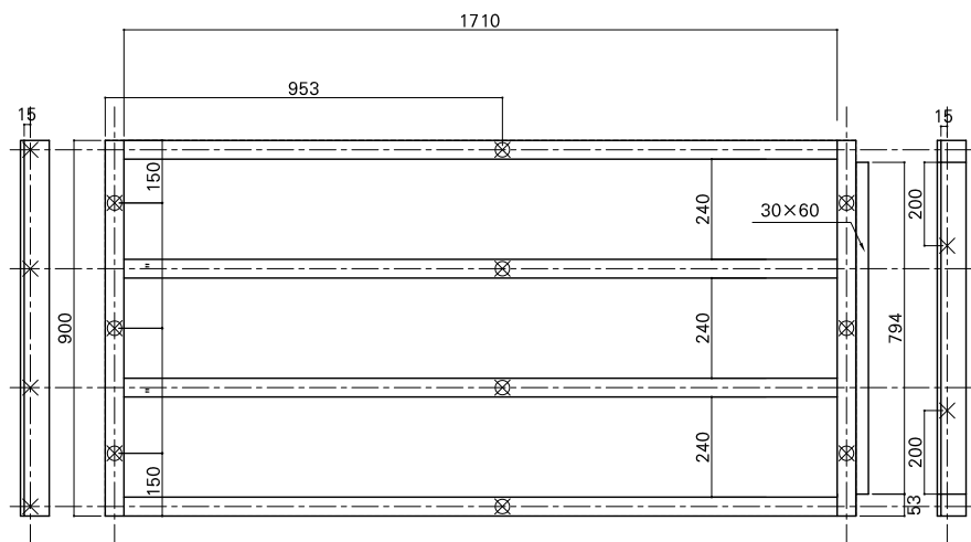
根太詳細図
