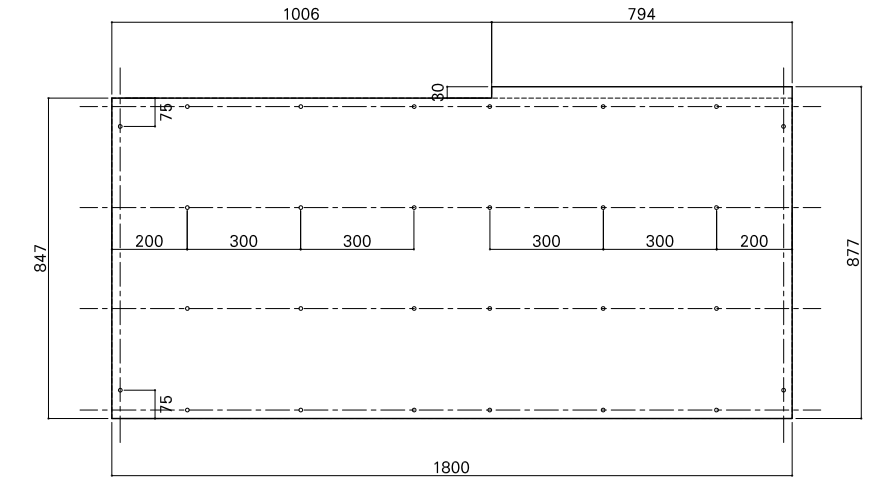
合板詳細図
