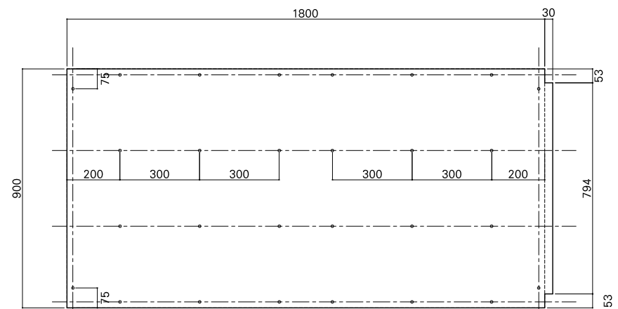
合板詳細図
